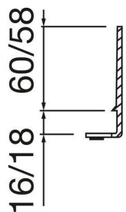
SEZ.A-A
